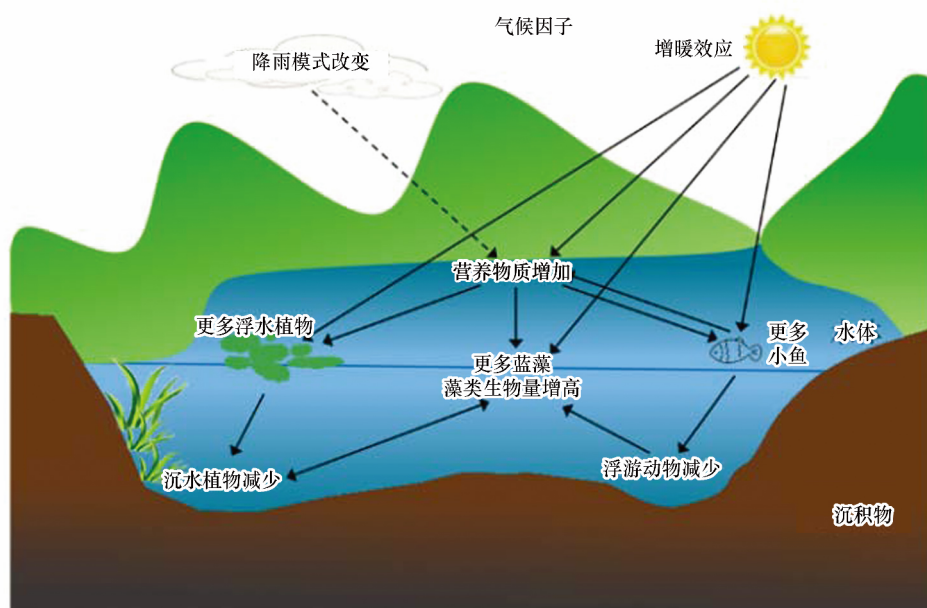
图1 气候变化对湖泊富营养化的驱动作用 (在 [5] 基础上改进)
