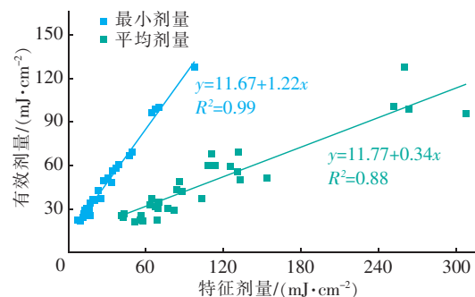
图9 紫外消毒器有效剂量与特征剂量之间的相关关系
