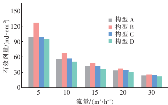
图 6 不同流量下各构型紫外消毒器的有效剂量
