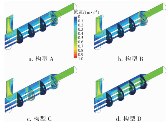
图 3 不同构型紫外消毒器中水流流速分布云图
