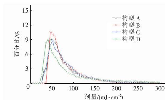
图5 不同构型紫外消毒器剂量分布曲线
